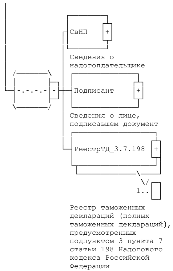
Рисунок 1. Диаграмма структуры файла обмена
