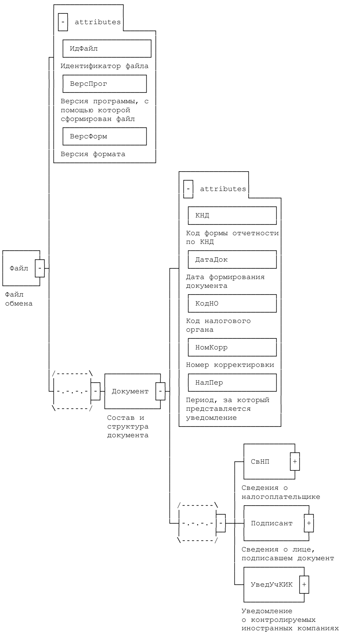
Рисунок 1. Диаграмма структуры файла обмена
